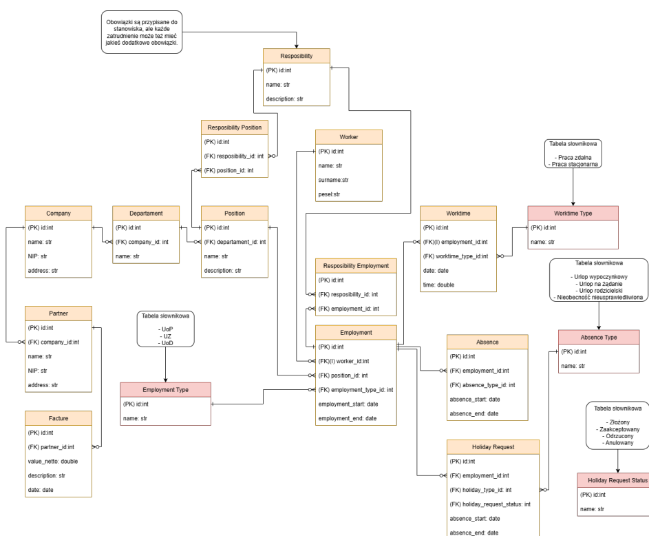
Rysunek 1: Diagram ERD systemu
